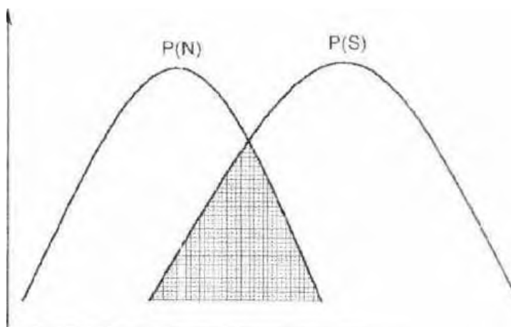
Рисунок 10.1 – Треугольник отказов
